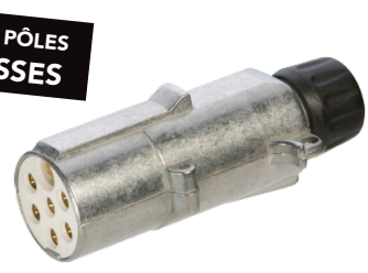
FICHE ALU 7 PÔLES 24S Ref. ERIC 211028 À cosses plates.
